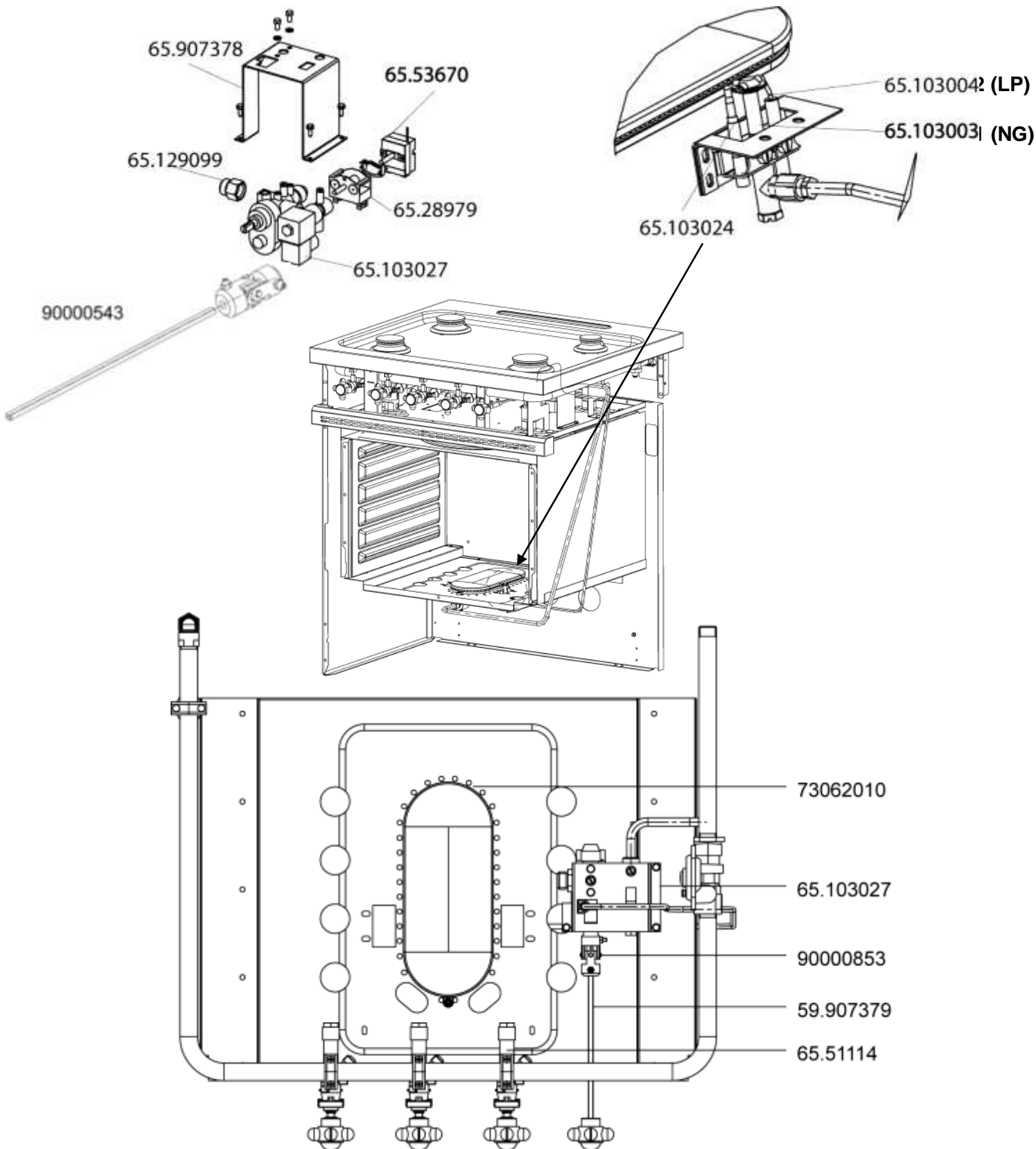
Détail A:
